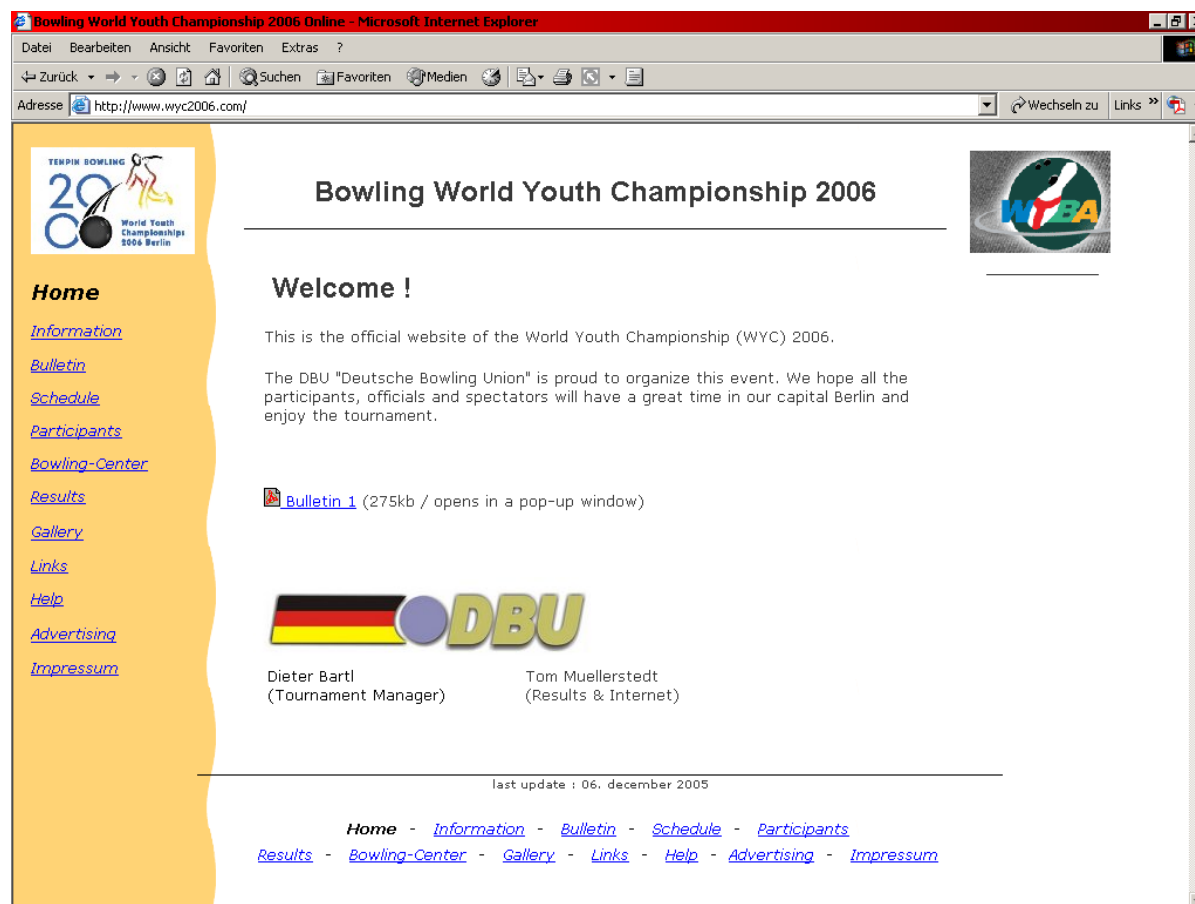
Abbildung 1: Hauptseite
